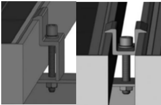
例子A: 压块夹紧式 Example A: Clamping
