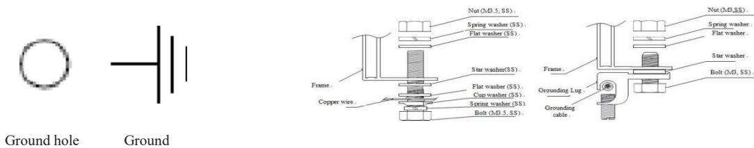
组件边框上接地孔示意
