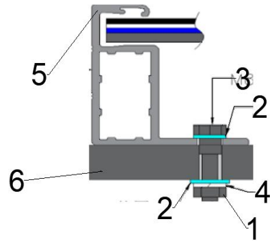
例子 B: 螺栓固定式 Example B: Bolting
